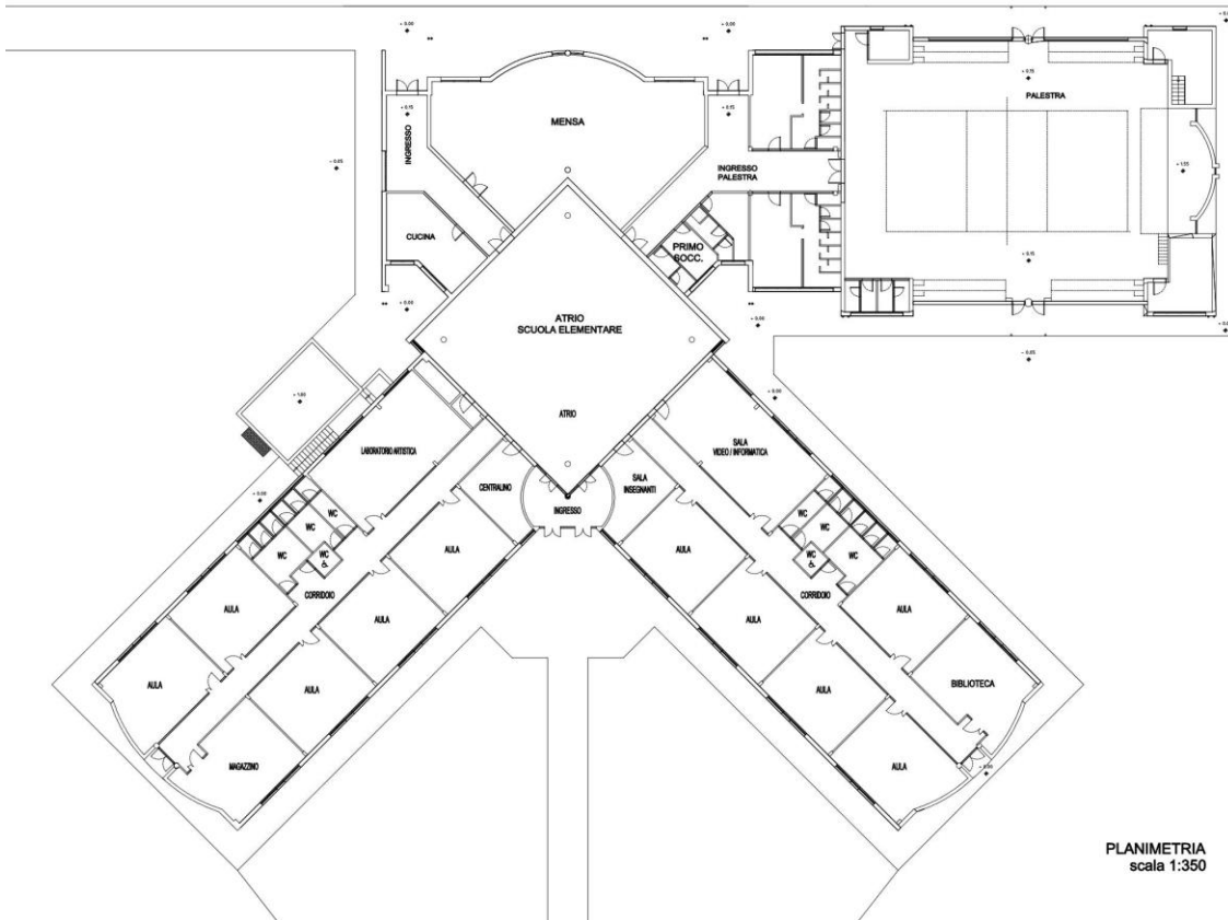
Planimetria della Scuola
